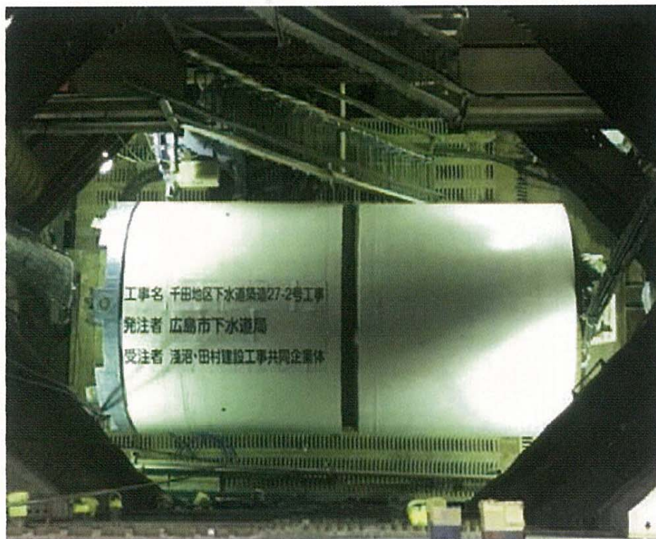
シールドマシン組立完了
