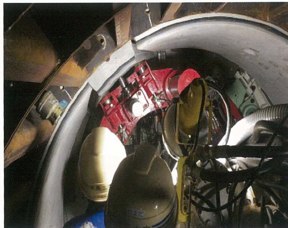
シールド坑内(セグメント組立)
