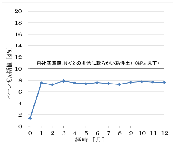
ベーンせん断値の経時変化
