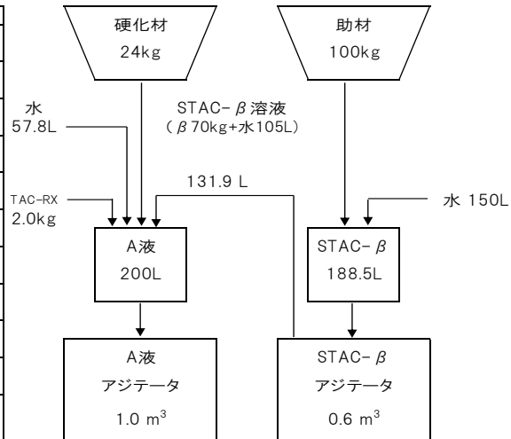
型式CSS-01 (寸法 L6.5m×W2.1m×H2.7m、電気容量 AC200V/25kW、空重量 5.3ton)
