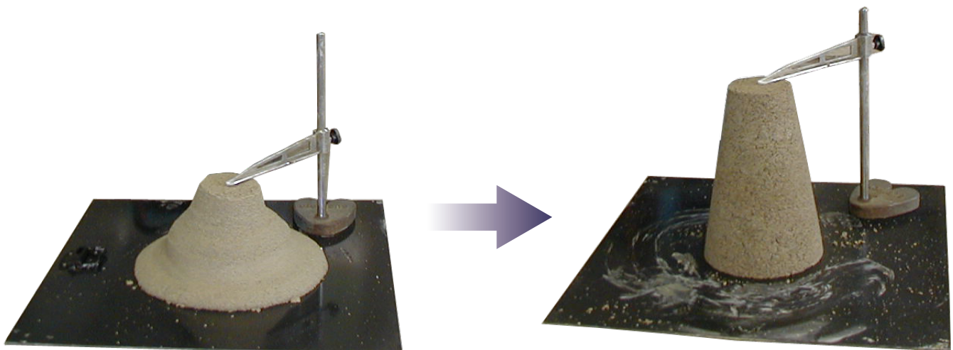
(気泡添加土砂スランプ試験)
