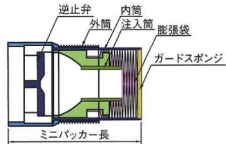
●ミニパッカー構造
